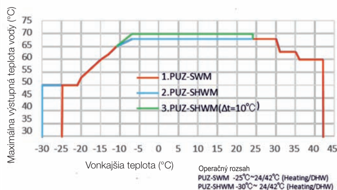
Graf závislosti výstupnej teploty vody od vonkajšej teploty
