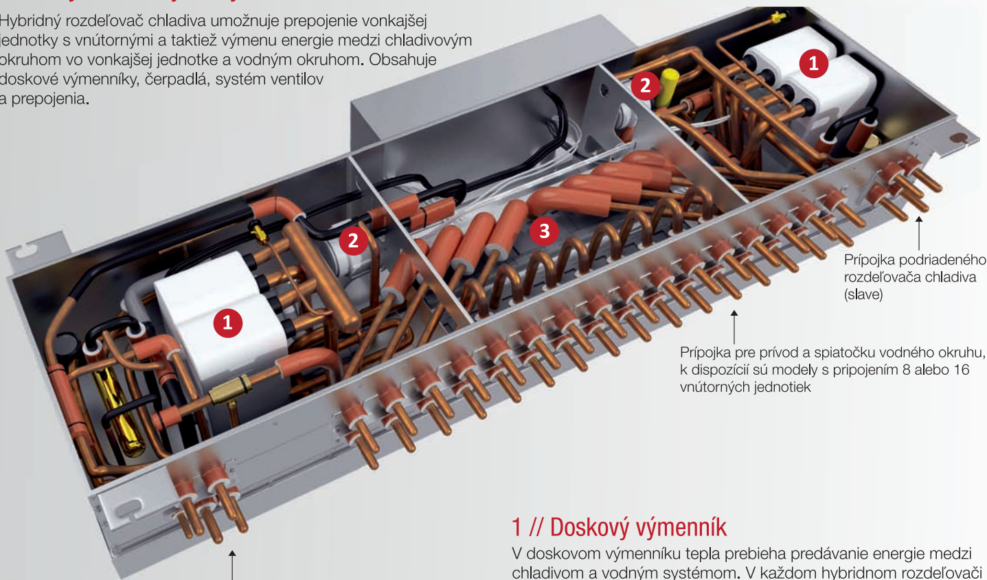
Prípojky pre chladivový okruh vonkajších jednotiek, externú expanznú nádobu a prívod vody
