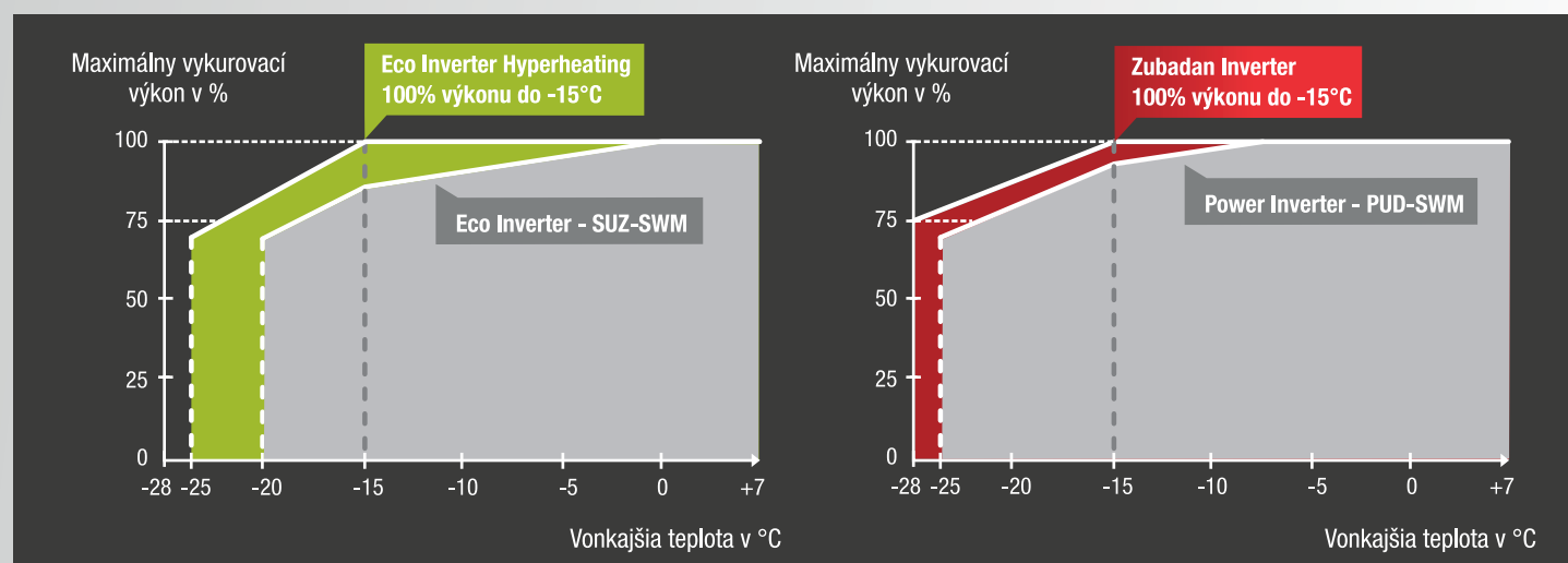
Graf závislosti výkonu od vonkajšej teploty
