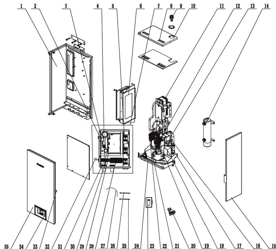
Seznam dílů GRS-CQ12Pd/NhH-M(I), GRS-CQ14Pd/NhH-M(I), GRS-CQ16Pd/NhH-M(I)
