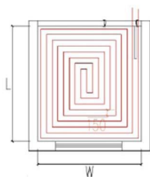
Smyčka ve tvaru čtvercové spirály (šnek, doporučeno)
